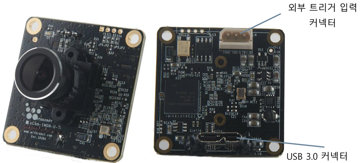
그림 1. oCam-1MGN-U-T 외형
