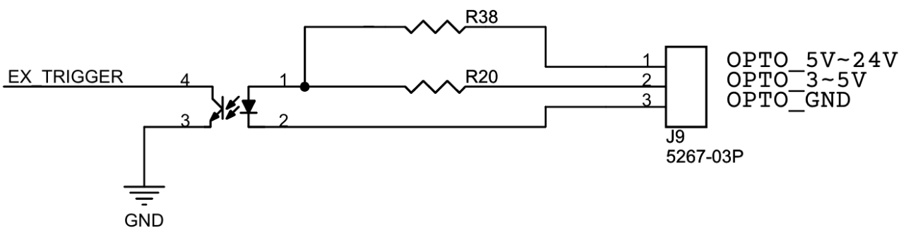
그림 7. 트리거 신호 입력 회로
